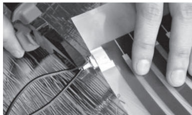
Рис. 12. Надежно зажмите провода в контактном зажиме
