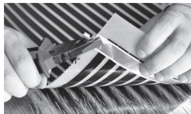
Рис. 6. Крепление контактного зажима к термопленке
