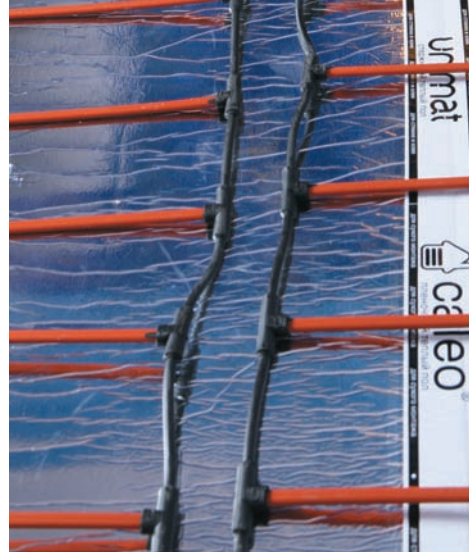
Рис. 10. Фиксация полос UNIMAT
