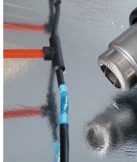
Рис. 13. Термоусадка соединительной гильзы техническим феном
