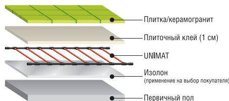
Рис. 25. Схема монтажа теплого пола UNIMAT под плитку/керамогранит
