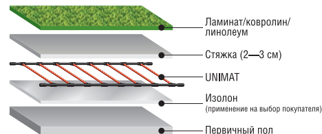
Рис. 23. Схема монтажа теплого пола UNIMAT под ламинат/ковролин/ линолеум
