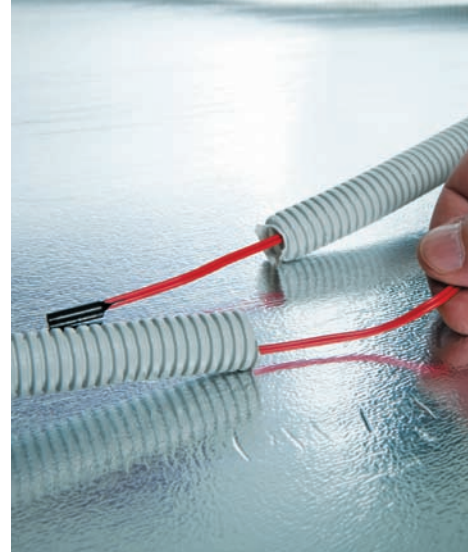
Рис. 18. Установка датчика температуры пола SF в гофрированную трубку (конец).
