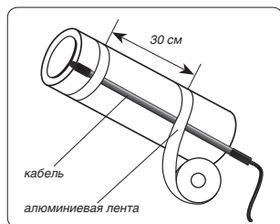
Рис. 1. Фиксация кабеля на трубе с помощью алюминиевой ленты
