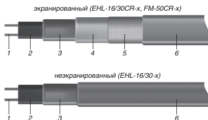
1. Токосоемущие медные жилы; 2. Нагревательная матрица с эффектом саморегуляции; 3. Первый слой изоляции; 4. Второй слой изоляции из полиолефина; 5. Экранирующая оплетка из луженой меди; 6. Защитная оболочка из полиолефина.
