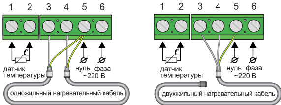
Рис.9 Схема подключения терморегулятора к 2-х проводной электросети
