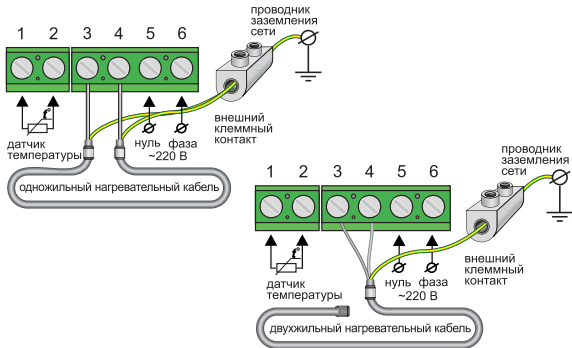
Рис. 10 Схема подключения терморегулятора к 3-х проводной электросети
