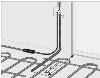
Рис.8 Монтаж датчика температуры пола
