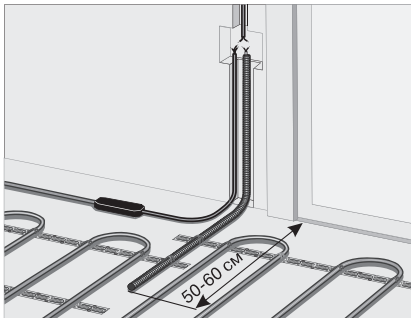
Рис. 62 Монтаж датчика температуры пола
